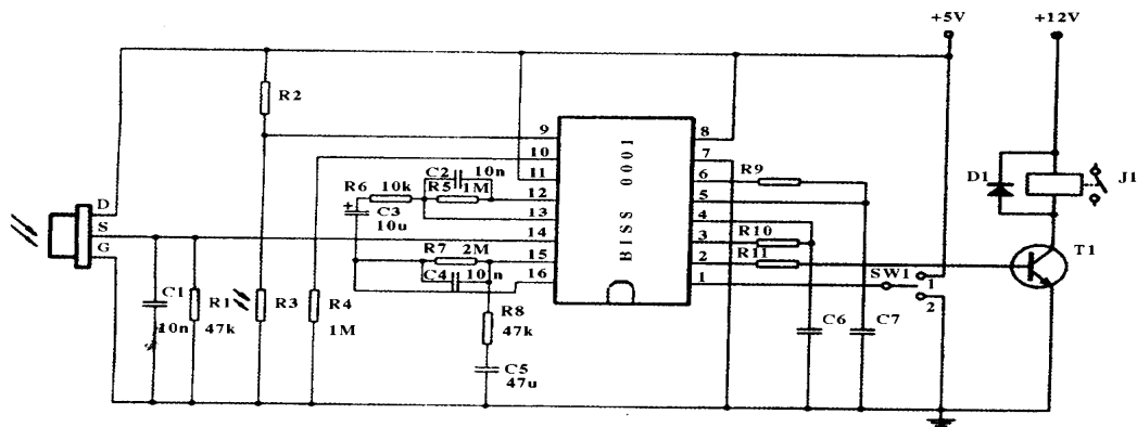
图5 执释由红外开关电路原理图
